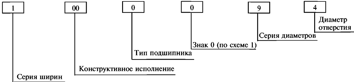
Подшипник 1000094 — радиальный шариковый однорядный
